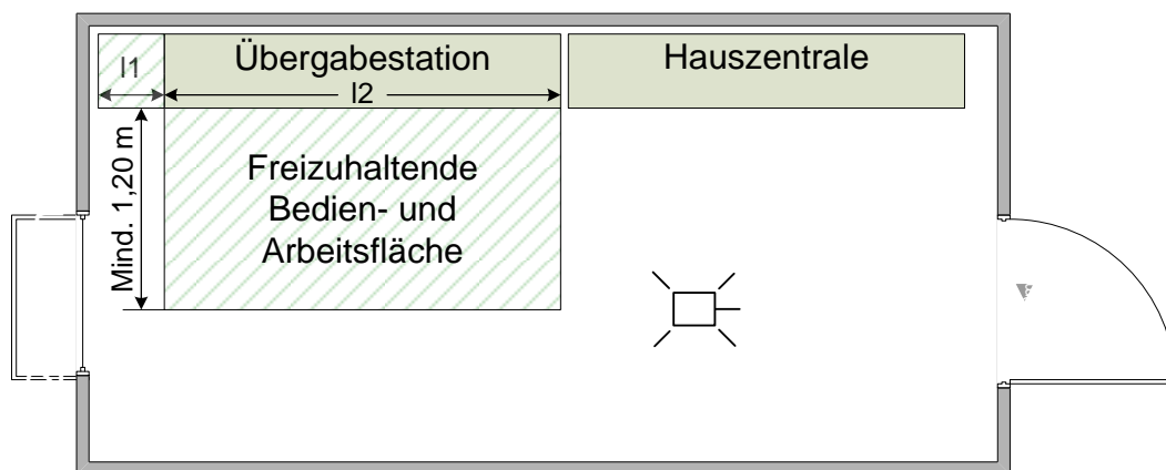
Abbildung 3: Hausanschlussraum
