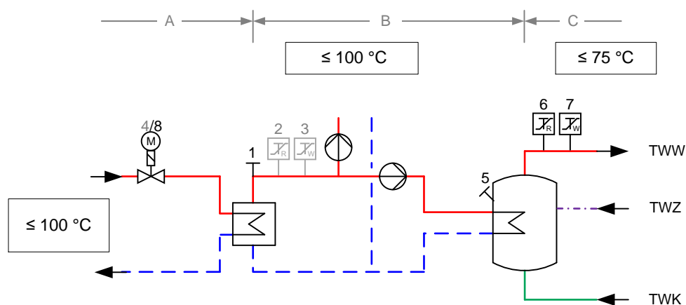
Abbildung zur Tabelle 8: Erforderliche sicherheitstechnische Ausrüstung nach Zeile 2; grau dargestellte Komponenten nicht erforderlich
