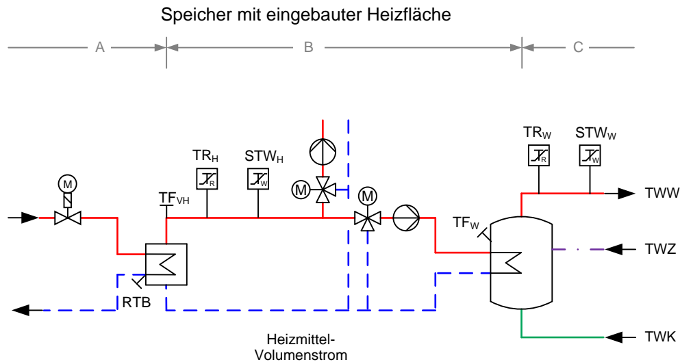
Abbildung 9: Hauszentrale-Trinkwassererwärmung; Prinzipschaltbild für den indirekten Anschluss
