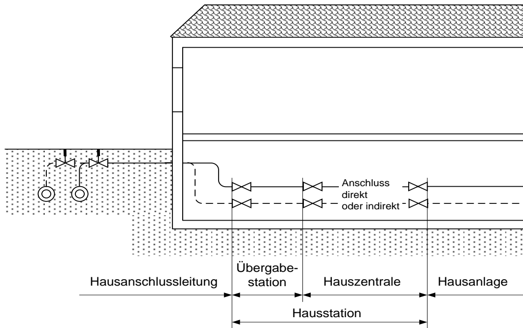
Abbildung 5: Hausanschlussleitung und Hausstation
