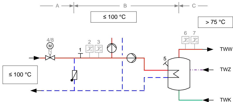
Abbildung zur Tabelle 8: Erforderliche sicherheitstechnische Ausrüstung nach Zeile 3; grau dargestellte Komponenten nicht erforderlich
