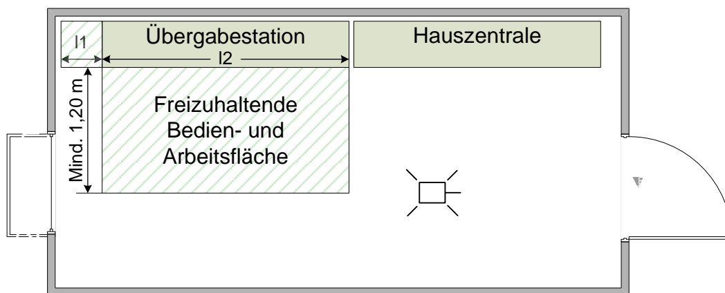
Abbildung 3: Hausanschlussraum
