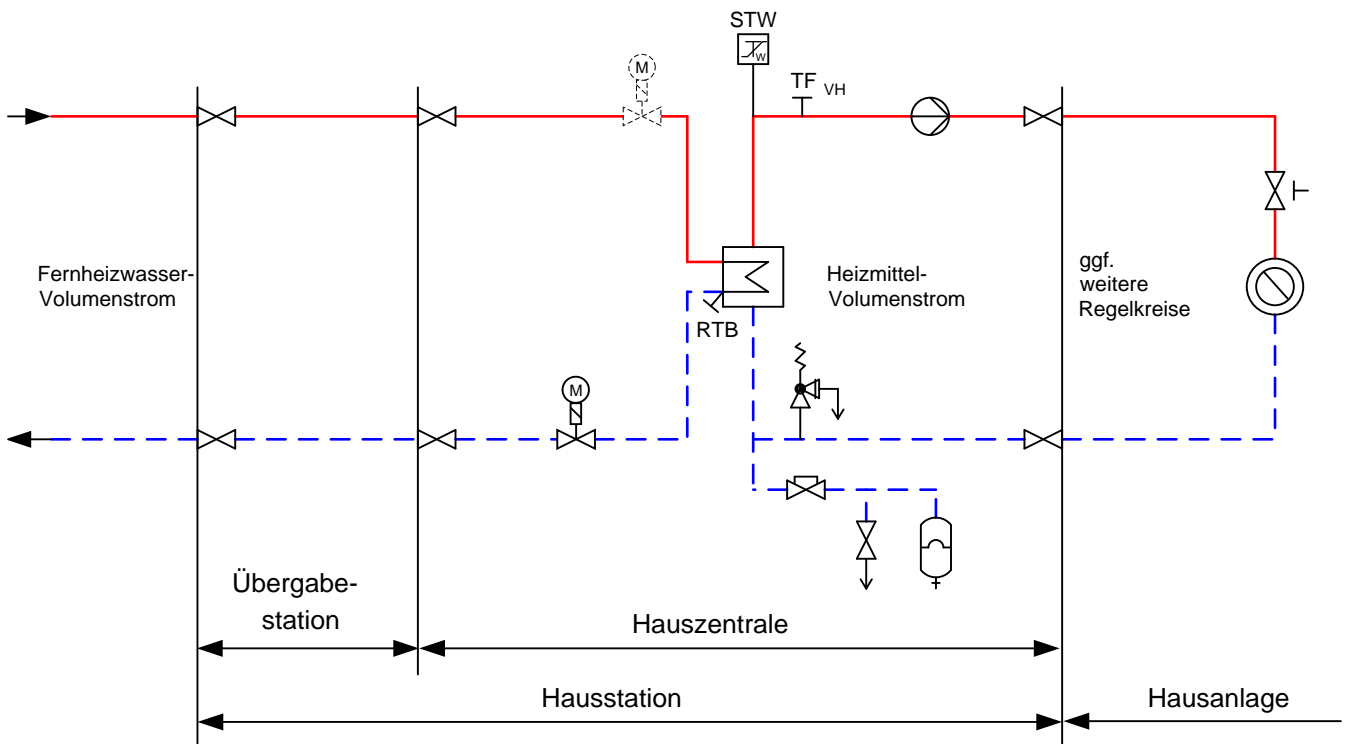
Abbildung 7: Hauszentrale-Raumheizung Prinzipschaltbild für den indirekten Anschluss
