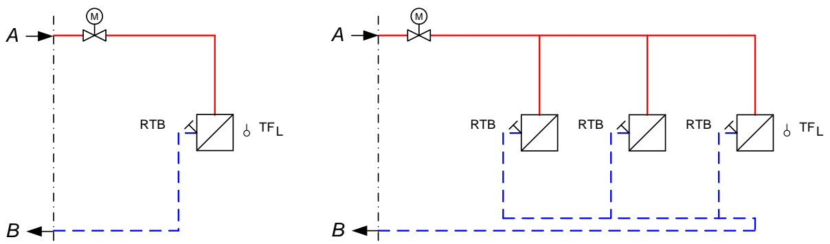
Abbildung 8: Hauszentrale-Raumluftheizung Prinzipschaltbilder für den indirekten Anschluss
