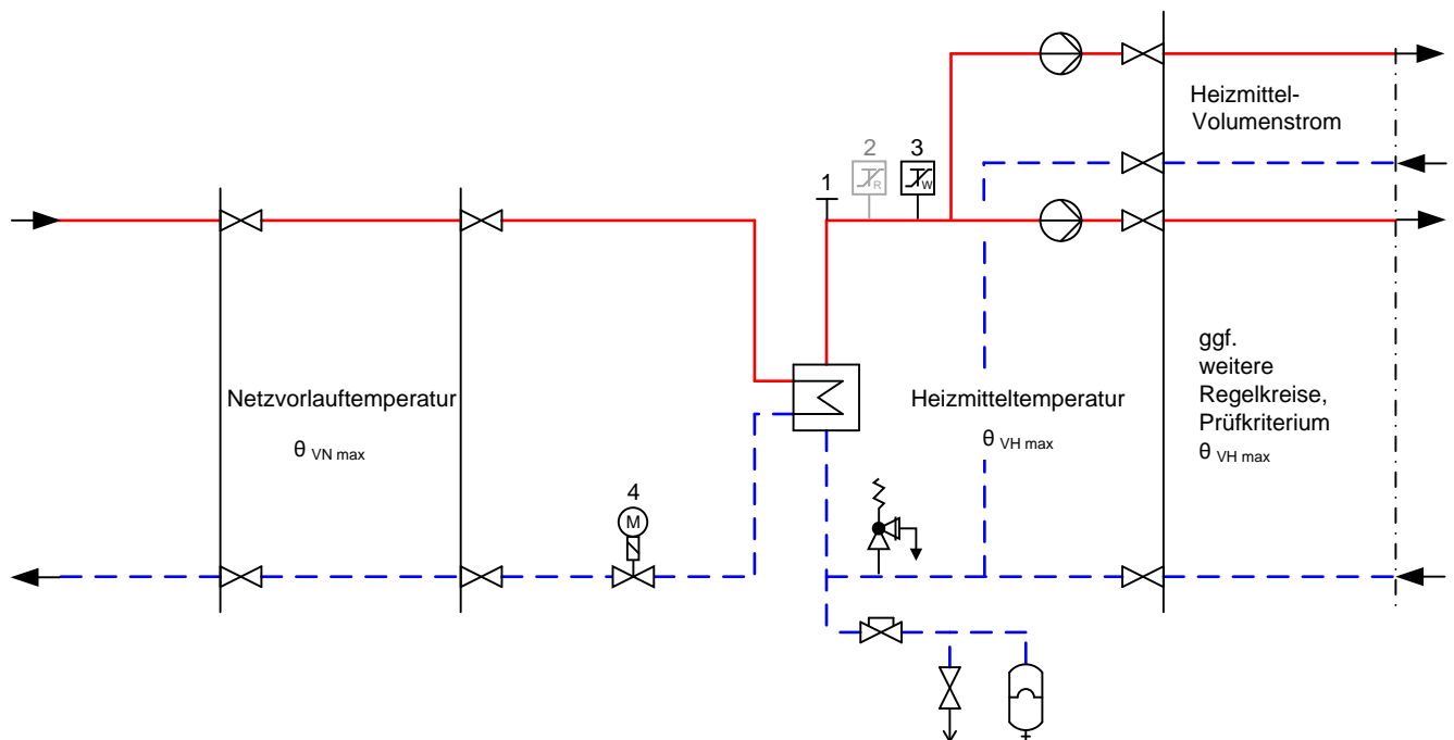
Abbildung zur Fehler! Verweisquelle konnte nicht gefunden werden.: Erforderliche sicherheitstechnische Ausrüstung nach Zeile 2;
