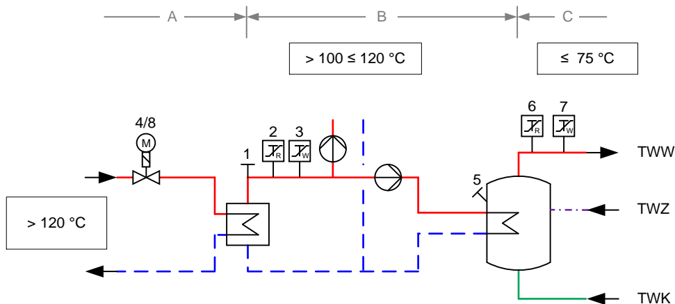
Abbildung zur Tabelle 8: Erforderliche sicherheitstechnische Ausrüstung nach Zeile 4
