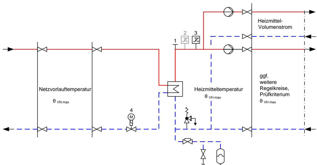
Abbildung zur Tabelle 6: Erforderliche sicherheitstechnische Ausrüstung; grau dargestellte Komponenten
