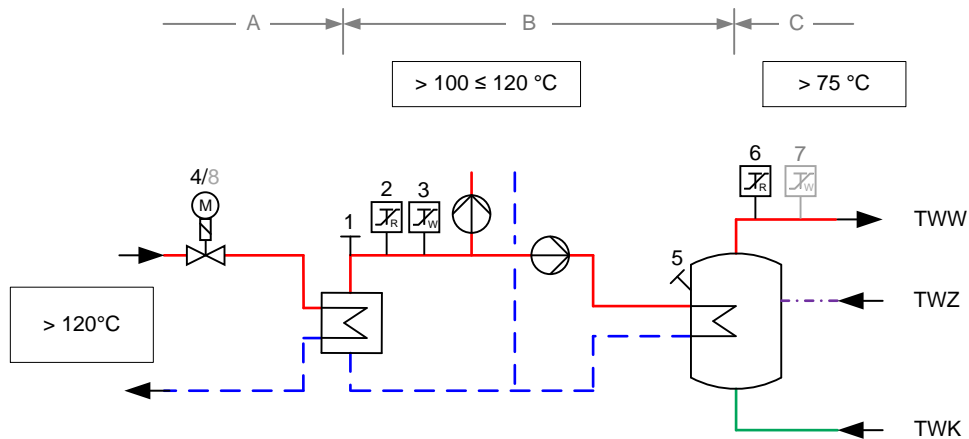
Abbildung zur Tabelle 8: Erforderliche sicherheitstechnische Ausrüstung nach Zeile 5; grau dargestellte Komponenten nicht erforderlich
