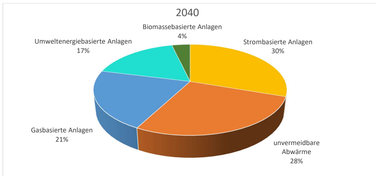
Abbildung 40: Thüringenweite Zusammensetzung der Fernwärmeerzeugung im Jahr 2040 nach Wärmemenge gemäß den Planungen der Fernwärmeversorgungsunternehmen (n=31) 220
