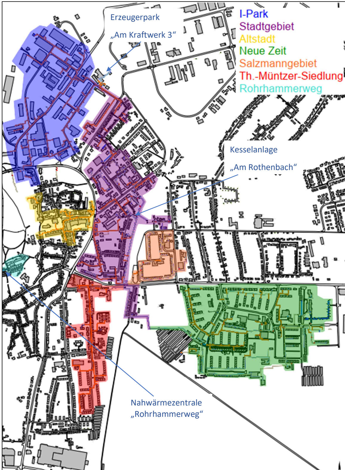
Abbildung 25: Netzkarte des Fernwärmenetzes der SEV
