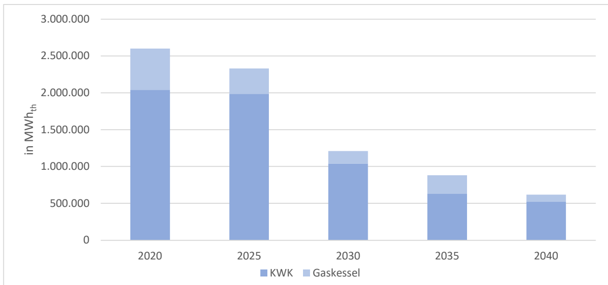
Abbildung 41: Entwicklung der Relevanz gasbasierter Anlagen, nach Wärmemenge (n=31)
