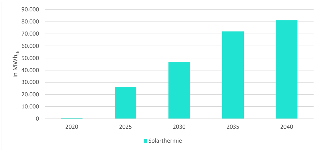
Abbildung 44: Angestrebte Entwicklung der Solarthermie (n=31)
